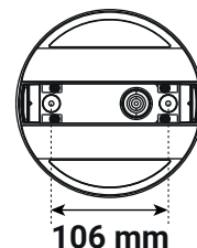
Schéma de fixation
