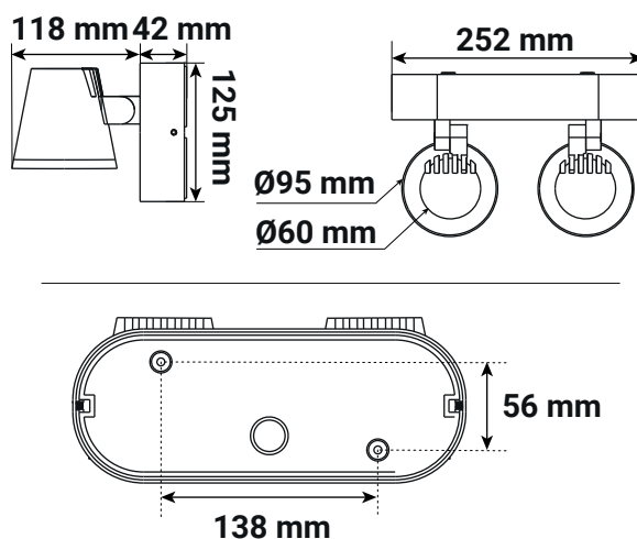
Schéma de fixation
