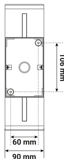
Schéma de fixation
