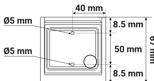
Schéma de fixation
