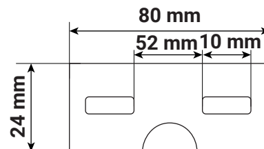
Schéma de fixation
