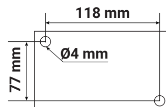
Schéma de fixation
