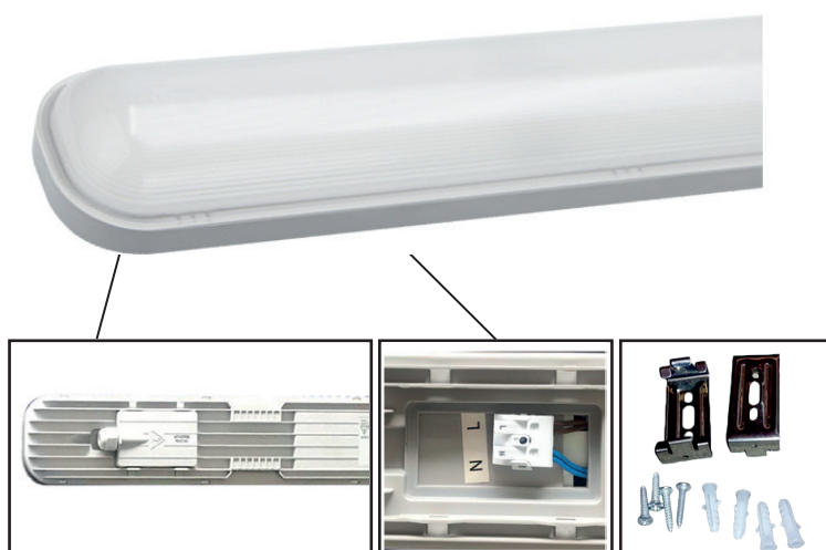
Boitier traversant
