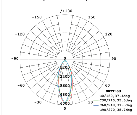
Courbe photométrique
